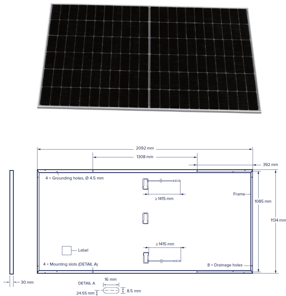
Слика 2 Предња и задња страна фотонапонског панела
