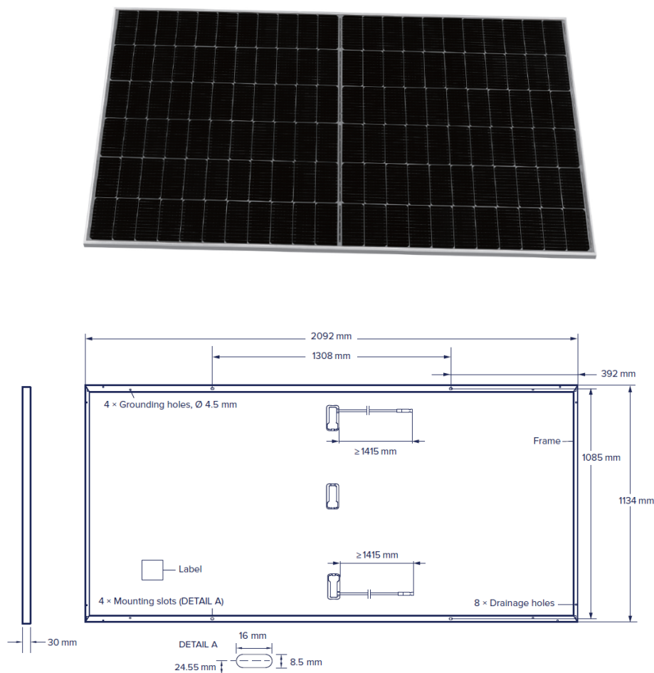
Слика бр. 2. Предња и задња страна фотонапонског панела
